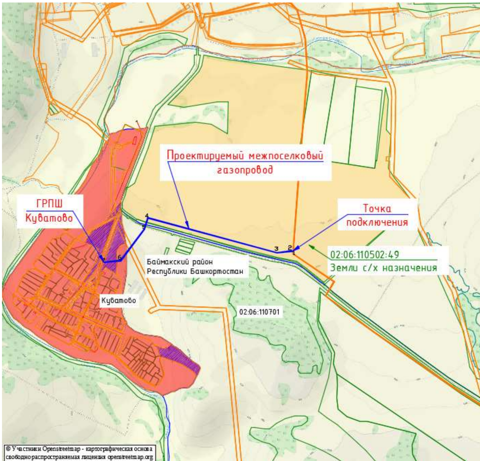
Рисунок 3.1 – Обзорная схема расположения проектируемого газопровода
